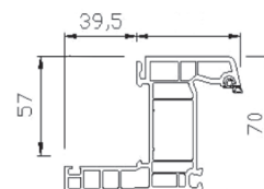
Réno aile de 39,5 mm
