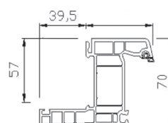
Réno aile de 39,5 mm
