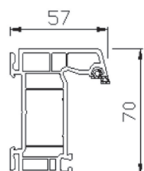
Sans aile avec double rainure
