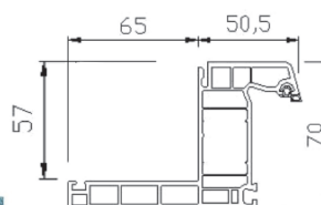
Réno aile de 65 mm
